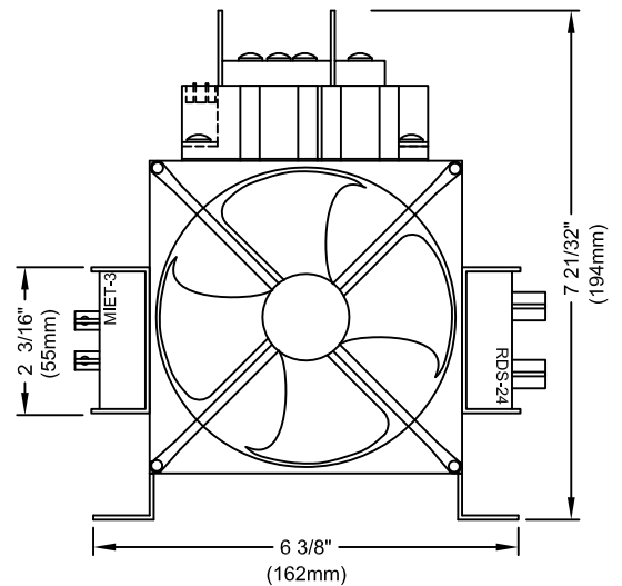
VUE DU BAS / BOTTOM VIEW
