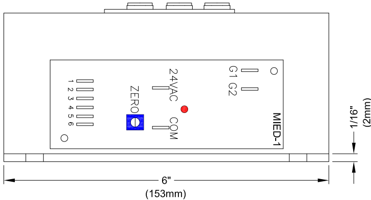
VUE DE CÔTÉ / SIDE VIEW
